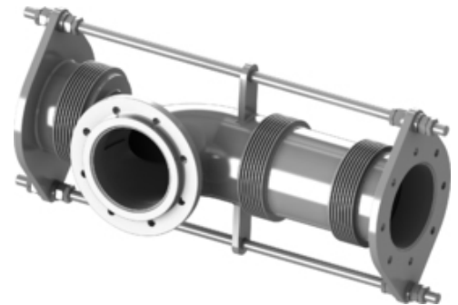
Megjegyzés| MPB típus - nyomáskiegyenlítő kompenzátor | 3D nézet
