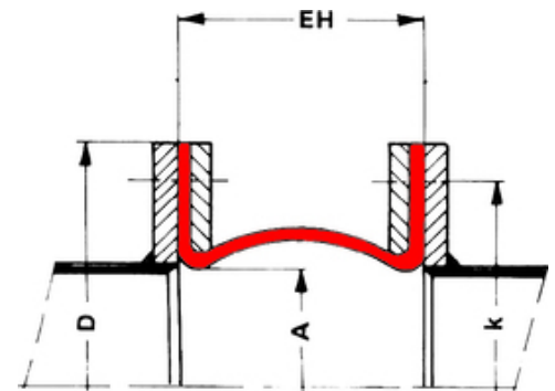
Megjegyzés | szövetkompenzátor - 32-es típus | méretrajz
