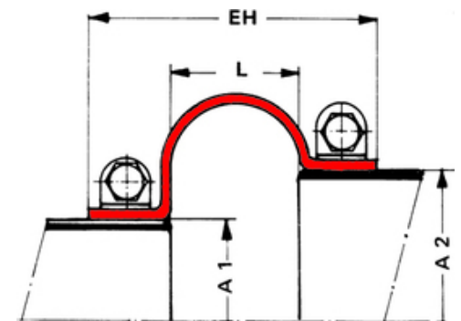
Megjegyzés | szövetkompenzátor - 16-os típus | méretraajz
