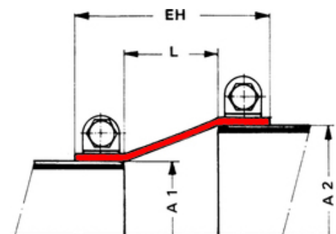
Megjegyzés | szövetkompenzátor - 15-ös típus | méretraajz
